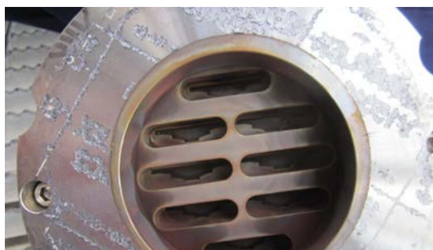
Fig. 7 La vanne a été démontée après 1 an d'utilisation sans dommages. Une vérification.
