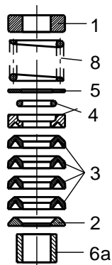
Vannes en acier inox DN15 et DN 20
