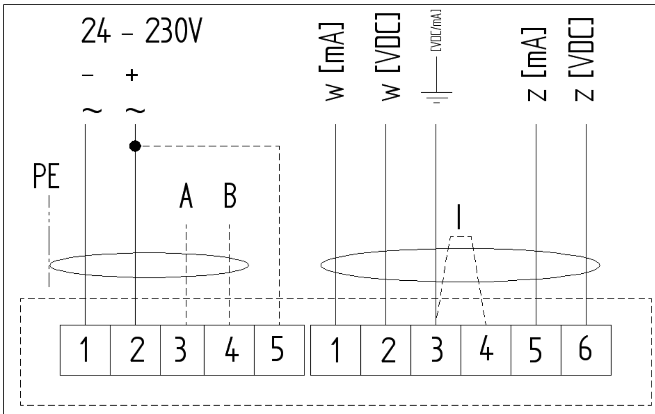
Schaltbild 2: DN25 bis DN80 mit Federrücklauf
